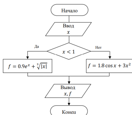
Блок-схема алгоритма
