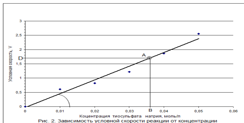
Рис. 2. Зависимость условной скорости реакции от концентрации
